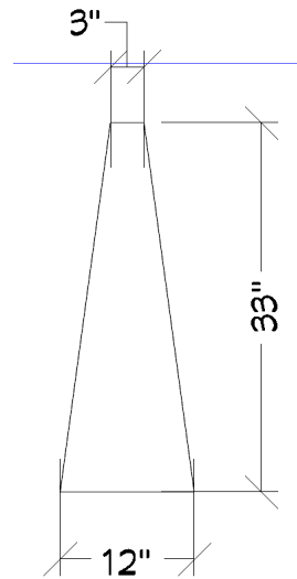
12" wedge
